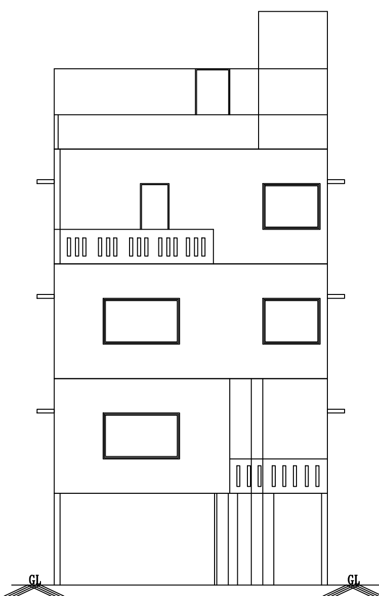
ELEVATION
