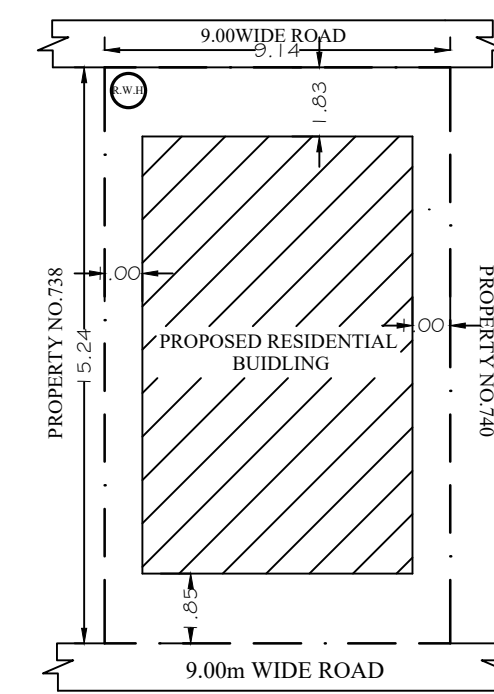
SITE PLAN 1:200
